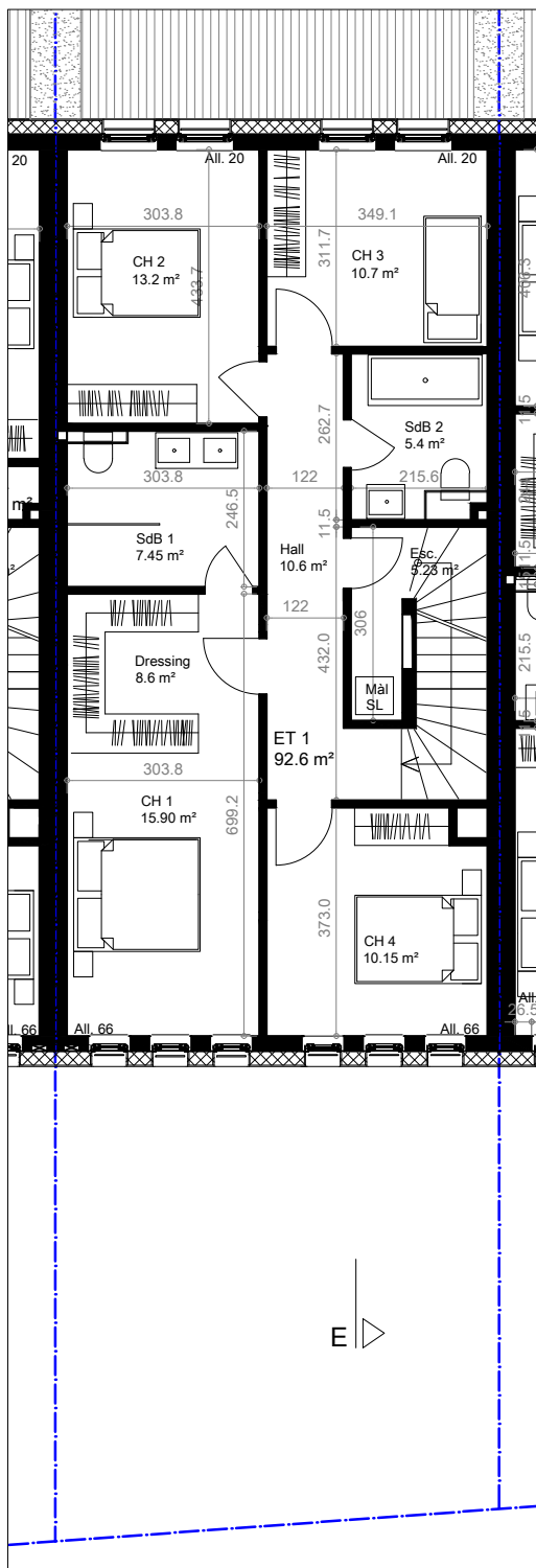
Maison 2 - NIVEAU +1
