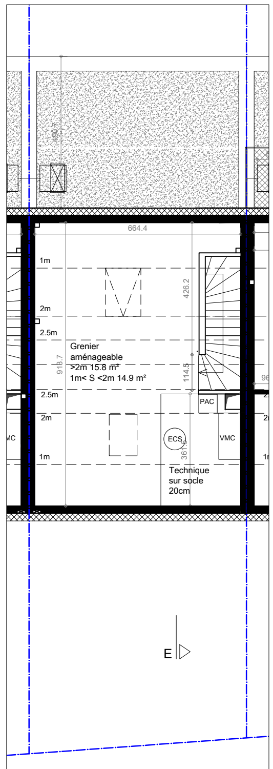
Maison 2 - NIVEAU +2
